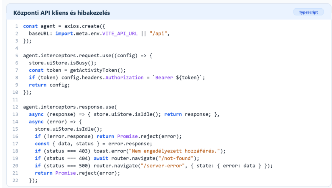
11. ábra: Központi API kliens és hibakezelés kódrészlete
